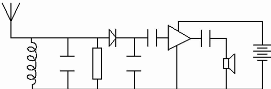
detektoros rádió kapcsolási rajza
